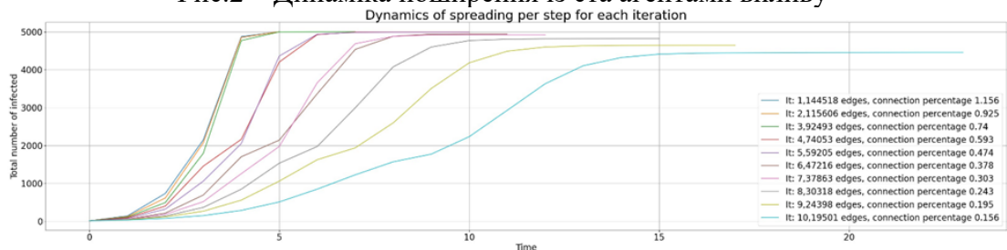
Рис.3 – Динаміка поширення із ста агентами впливу в одній групі
