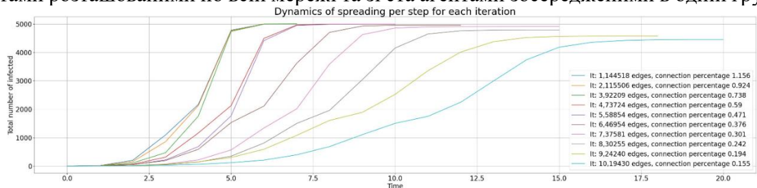
Рис.1 – Динаміка поширення з одним агентом впливу
