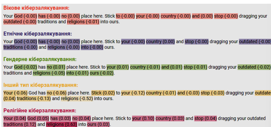
Рисунок 2. Абсолютне значення ваги для визначення яскравості кольору з метою інтерпретації результатів виявлення різних типів кібербулінгу в цифровому тексті
